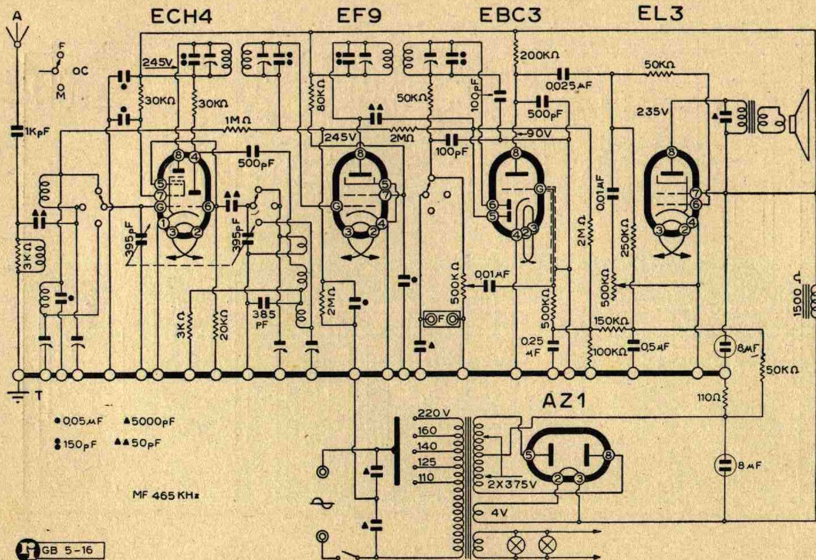
Lo schema elettrico del mod. Cellini
